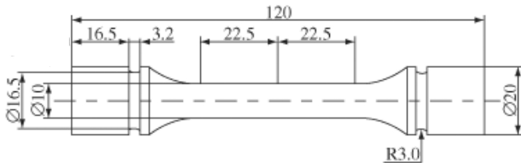
Rys.1. Próbkę do badania wytrzymałości na rozciąganie grafitu (wymiar w mm)
